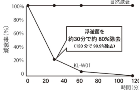
浮遊菌除去性能
